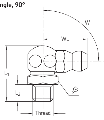
Angle, 90°
